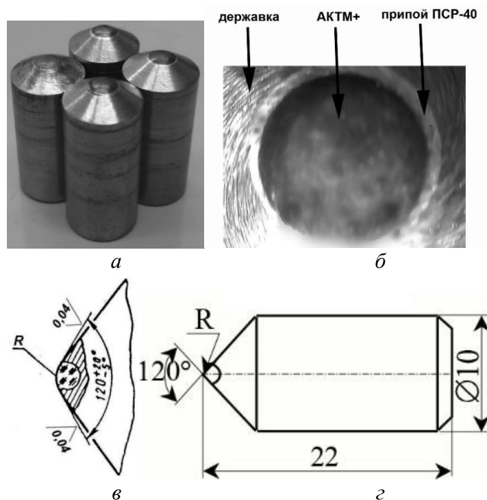
Рис. 3. Общий вид и основные размеры изготовленных износостойких наконечников
