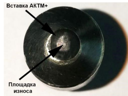
Рис. 6. Внешний вид выглаживателя, оснащенного алмазным композитом АКТМ+, после 95000 м пути
