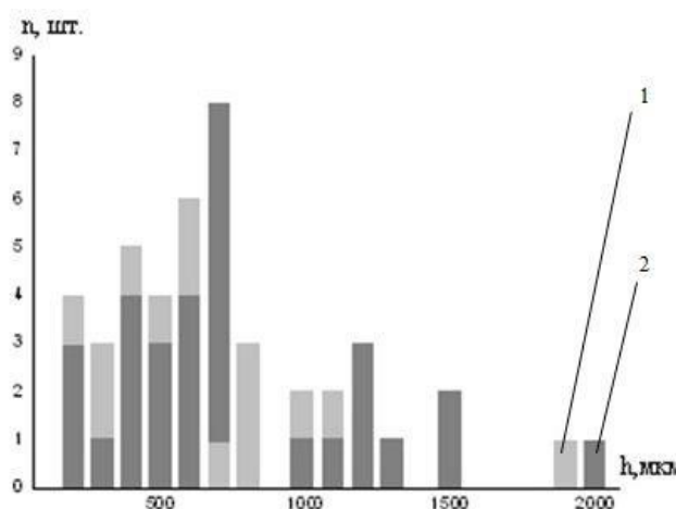
Рис. 6. Сравнительное распределение толщины частиц шлама, полученного в результате обработки коронок: 1 – со вставками АКМ; 2 – со вставками АПКМ+
