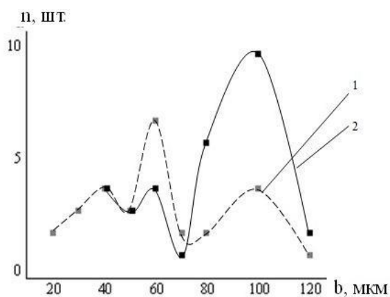
Рис. 5. Высота выступания алмазных зерен из матрицы: 1 – коронка, оснащенная вставками АКМ, 2 – коронка, оснащенная вставками АПКМ+
