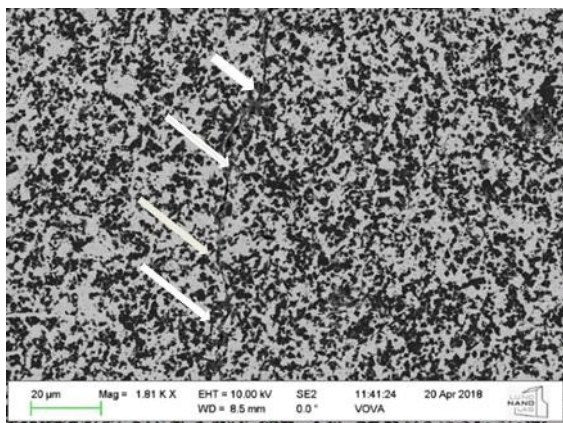
Рис. 5. Мікрострутури зразків, отриманих за допомогою скануючого електронного мікроскопа Hitachi SU8010 Cold Field Emission для неармованого мікрОВОЛОКОНАМИ зразка, спеченого за температури 1610 °C (а), та для армованого 5% мікрОВОЛОКОН SiC зразка, спеченого за температури 2025 °C (б)
