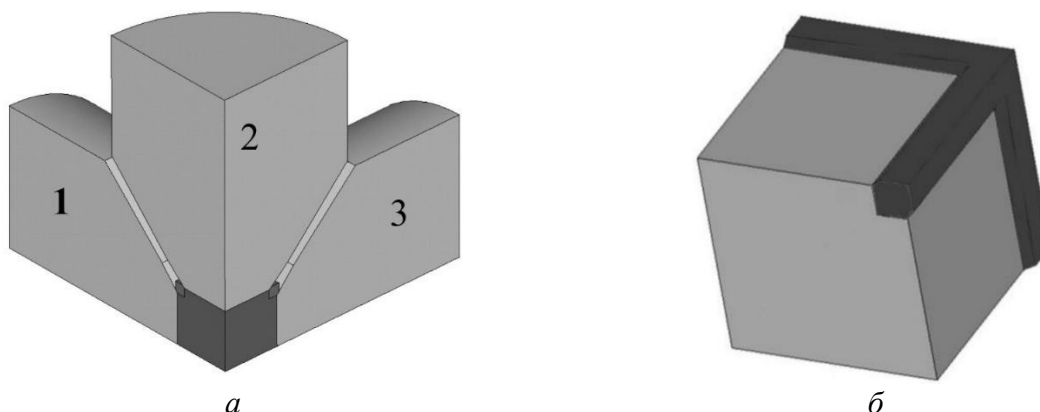
Рис.2. Процес навантаження пірофілітового куба при стисненні між пуансонами шестипуансонного АВТ: а – рух пуансонів на першій стадії моделювання.; б – утворення прокладки стиснення на першій стадії моделювання
