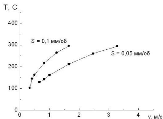
Рис. 5. График изменения температуры в зоне резания T при обработке сплава алюминия (а), латуни (б) в зависимости от скорости резания v
